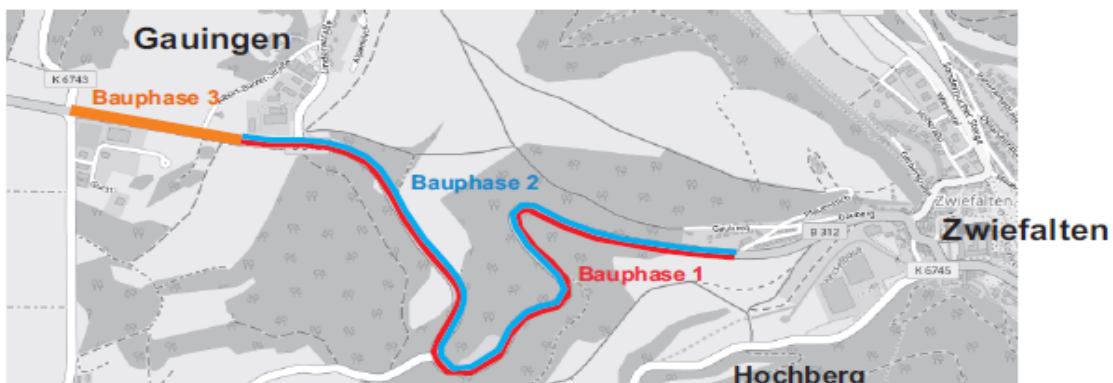
Regierungspräsidium Tübingen, Referat 47.1, Straßenbau Nord B 312, Fahrbahndeckenerneuerung Zwiefalter Steige Plan 1 Übersichtsplan überörtliche Umleitung und Bauphasen
